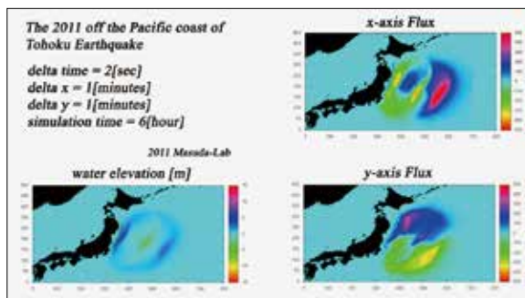
東北地方太平洋沖地震津波の再現シミュレーション
