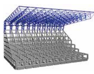
図 1 スタジアムの詳細解析モデル
