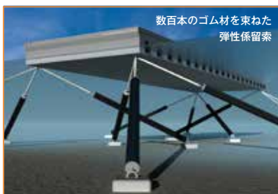
大型浮体を固定する弾性係留システムの設計
